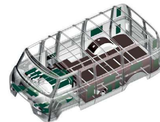
Пакет вибро- и шумоизоляции по всему кузову и специальные подушки крепления кузова
